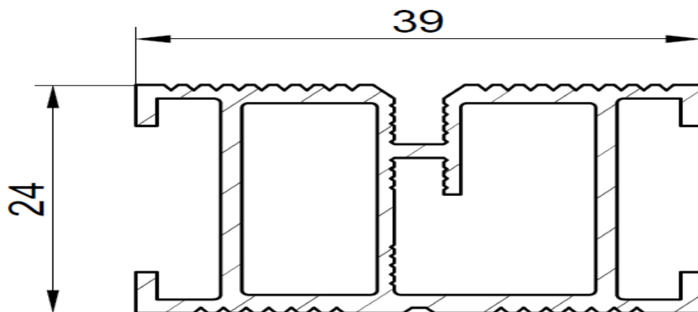
Rys. 4 Rysunek legara aluminiowego
