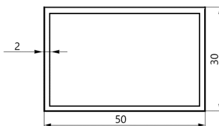
Rys. 5 Rysunek legara aluminiowego
