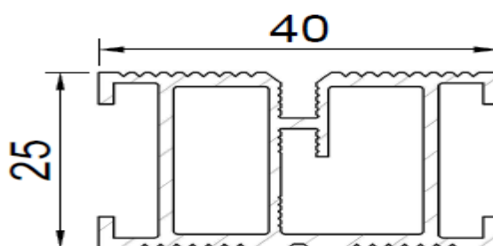
Rys. 1 Rysunek deski
