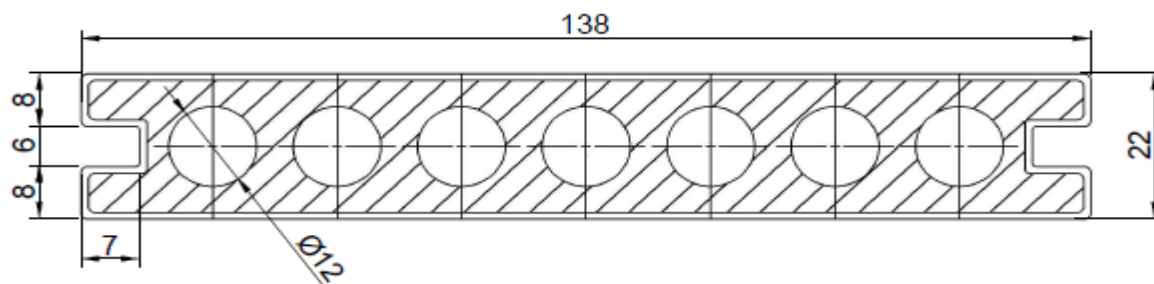
Rys. 1 Rysunek deski
