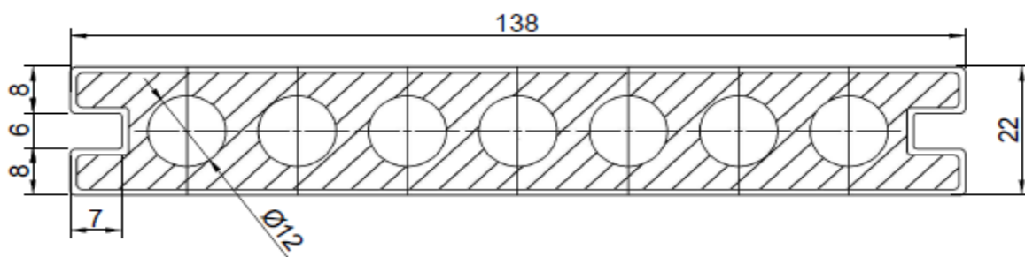
Rys. 1 Rysunek deski
