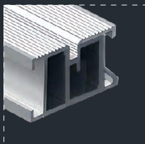
Алюминиевая лага 40 x 25 x 3000 / 4000 мм
