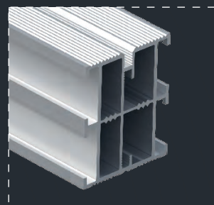
Алюмінієва лага 40 x 50 x 3000 / 4000 мм
