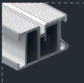
Алюмінієва лага 40 x 25 x 3000 / 4000 мм
